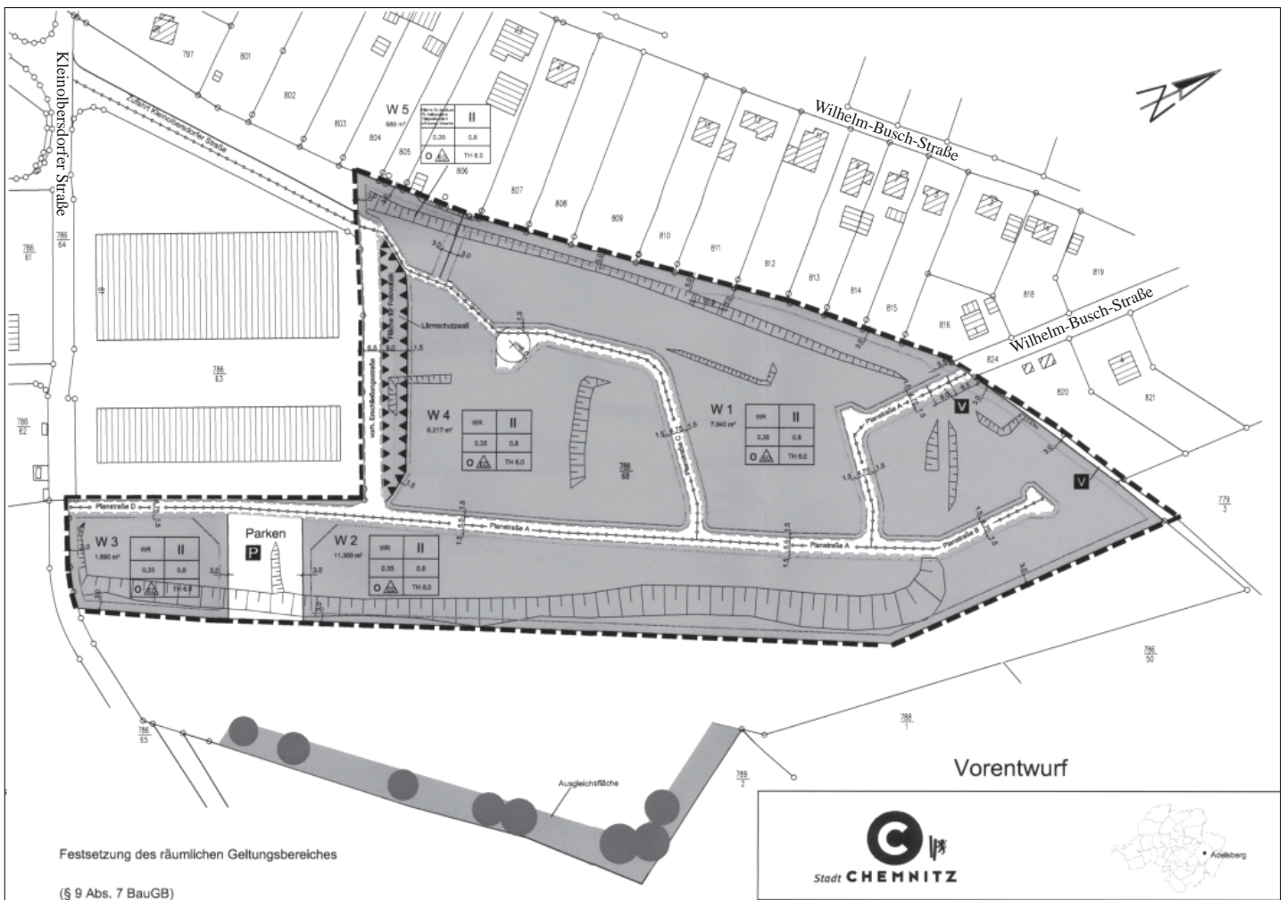
Vorentwurf des Vorhabenbezogenen Bebauungsplans für das Baugelände Adelsberg Kleinobersdorfer Straße/Wilhelm-Busch-Straße.
